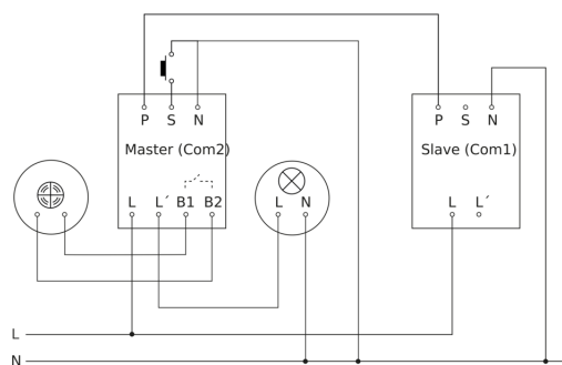
Diagrama electrónico interconexión maestro-esclavo
