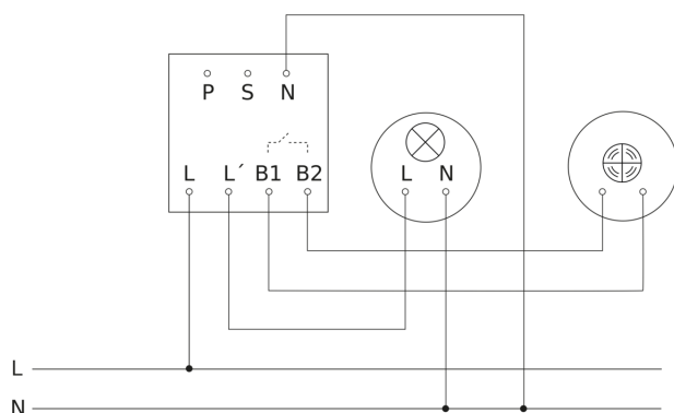
Diagrama electrónico maestro
